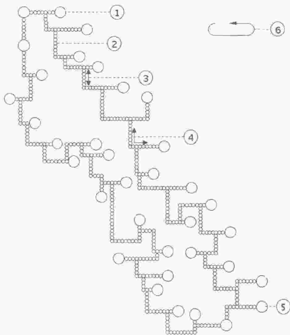
1. 色粒信息胶子, 2. 色粒信息胶子中迷粒子个数, 3. 迷粒子连接位置及个数, 4. 迷粒子信息确认连接方向, 5. 分裂旁系原体肌肽线粒体端向色粒信息胶子, 6. 色粒信息胶子信息解码标识, 为正向解码标识。
